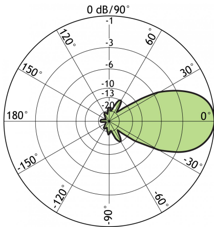
H-PLANE: Outer ring 11 dBd
