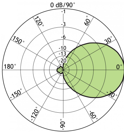
H-PLANE: Outer ring 6 dBd
