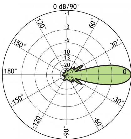
H-PLANE: Outer ring 15 dBd
